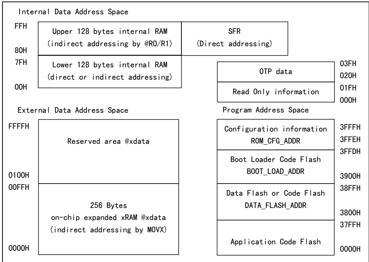
图 6.1 存储器结构图
