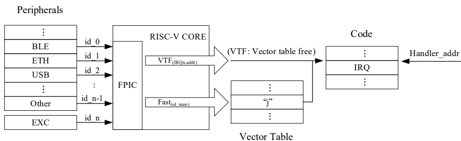
图 3-2 可编程快速中断控制器示意图
