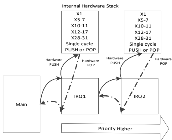
图 3-1 压栈示意图
