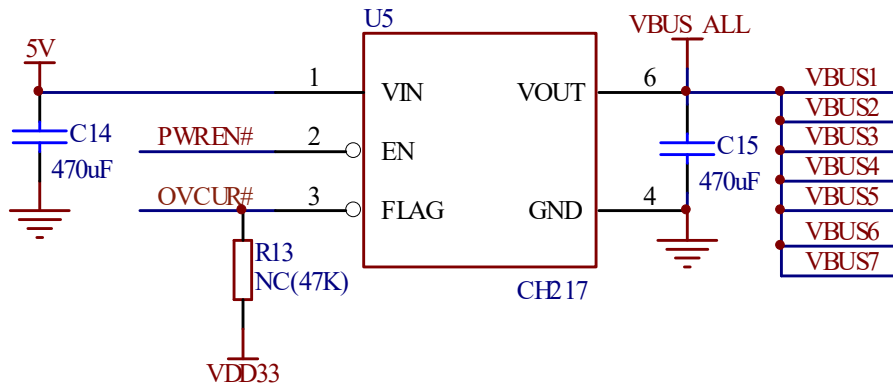
图 5-2 整体过流检测和独立电源控制
