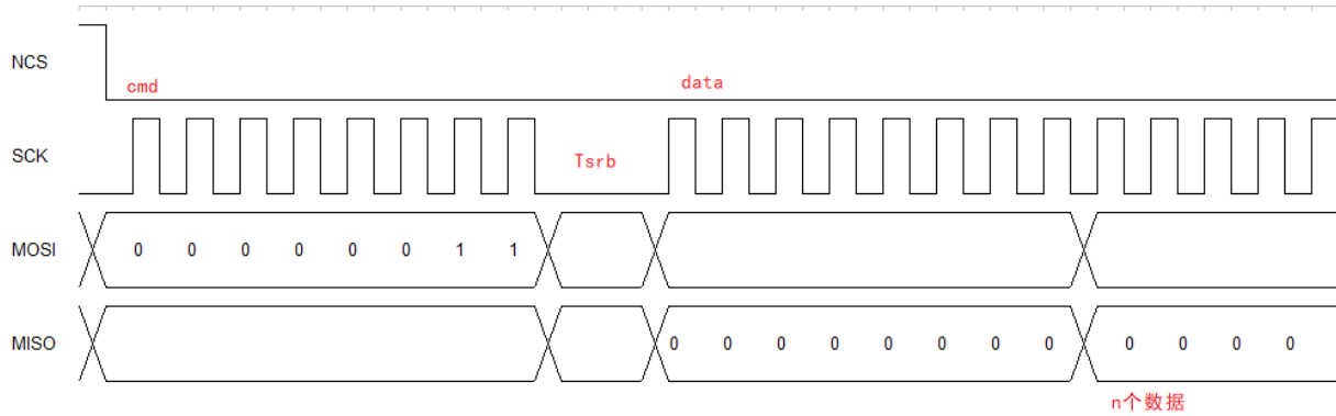
图 6-5 读 RX 缓冲区指令时序图
