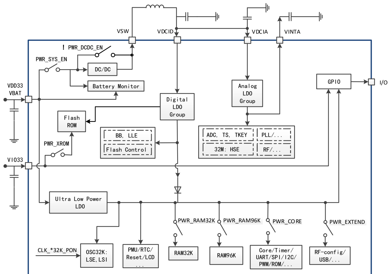
5-1 电源系统
