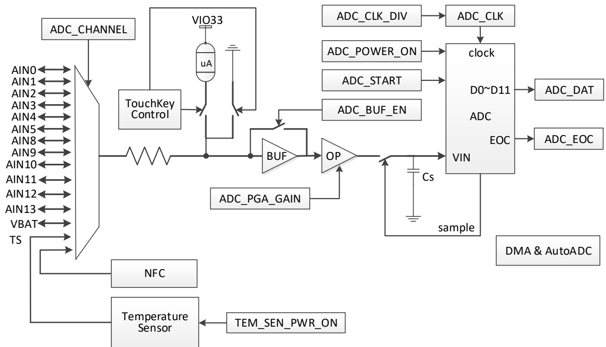
图 15-1 ADC 结构图
