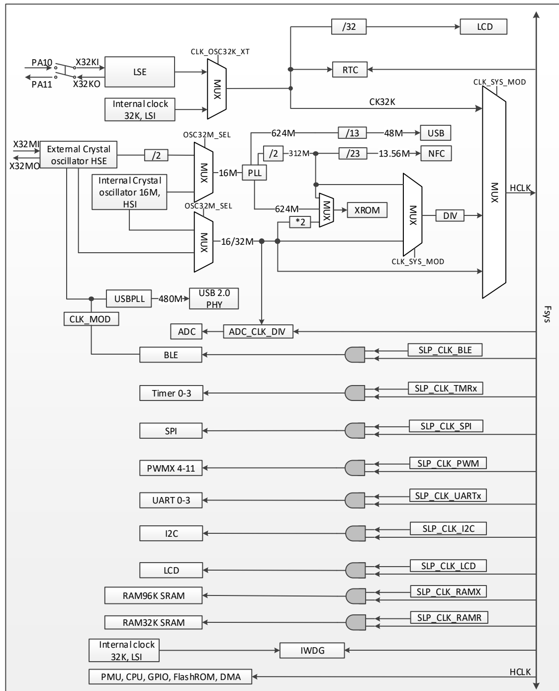
图 6-1 时钟树框图
